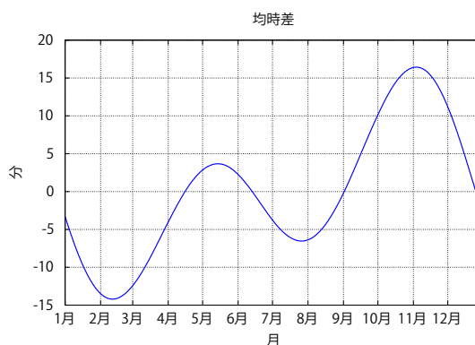
図 2: 均時差
