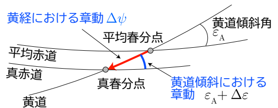
図 4: 黄経における章動と黄道傾斜における章動
